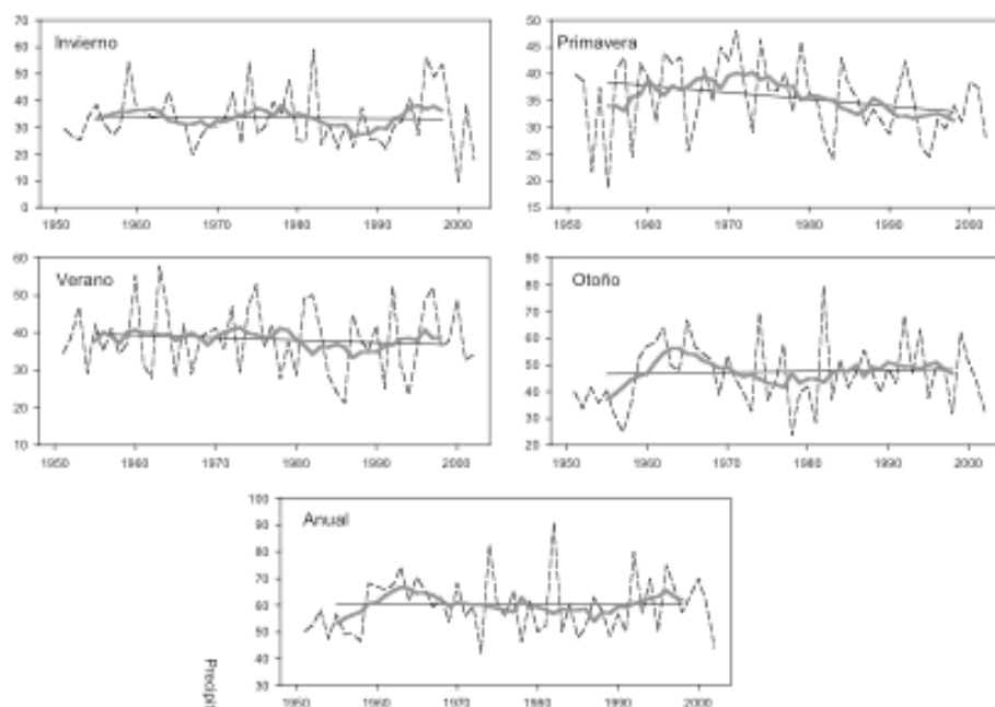
Figura 8. Evolución del valor máximo estacional y anual (1951-2001). Línea negra discontinua (precipitación observada), línea gris (filtro de 9 años). La línea de tendencia se obtiene mediante el ajuste por mínimos cuadrados a partir de los datos filtrados.
