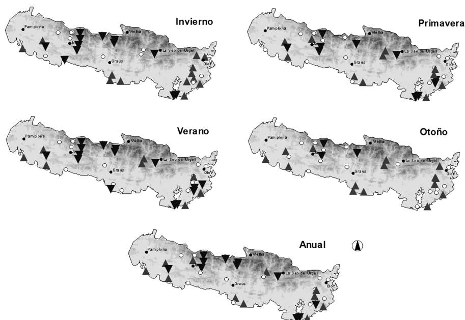
Figura 5. Distribución espacial de las tendencias en el número de días de precipitación estacional y anual (1951-2002). Triángulos: tendencia positiva y significativa. Triángulos invertidos: tendencia negativa y significativa. Círculos: Tendencia no significativa.
