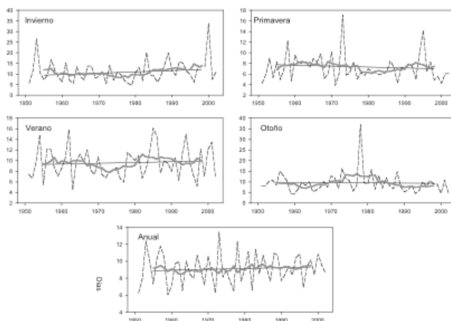
Figura 10. Evolución de la duración media de las rachas secas (1951-2001). Línea negra discontinua (promedio de duración de las rachas secas), línea gris (filtro de 9 años). La línea de tendencia se obtiene mediante el ajuste por mínimos cuadrados a partir de los datos filtrados. Figure 10. Evolution of the seasonal and annual average duration of dry spells (1951-2001). Black line (observed number of days), gray line (low pass filter of 9 years). The trend line has been obtained by means of regression analysis by means of filtered data.
