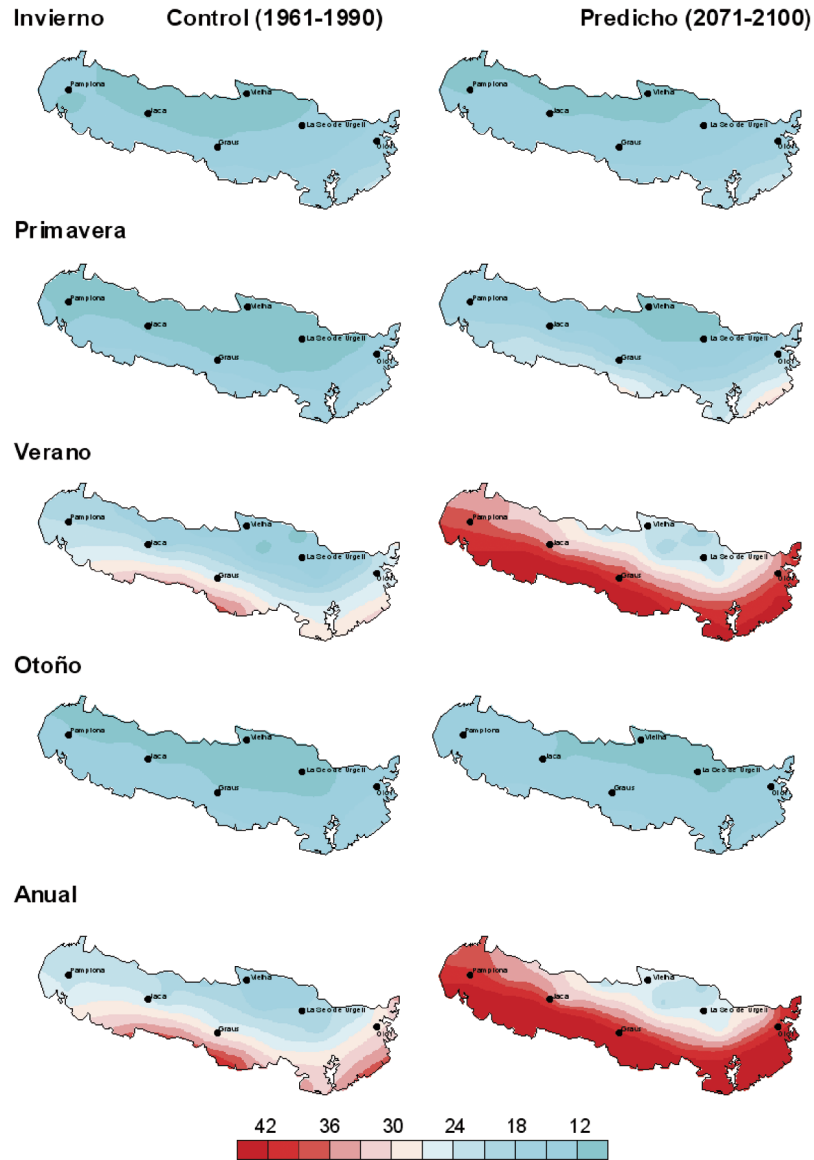
Figura 17: Distribución espacial del promedio de duración en días de la racha seca máxima registrada cada año. Modelo RCAO, SMHI. Periodo de control (1961-1990) y escenario A2 (2071-2100).
