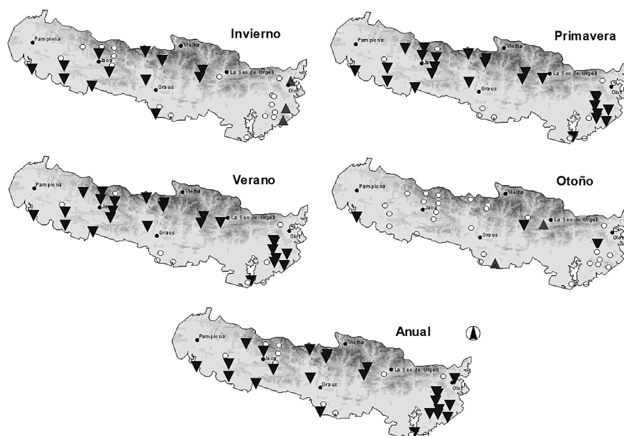
Figura 3. Distribución espacial de las tendencias en el volumen estacional y anual (1951-2002). Triángulos: tendencia positiva y significativa. Triángulos invertidos: tendencia negativa y significativa. Círculos: Tendencia no significativa.
