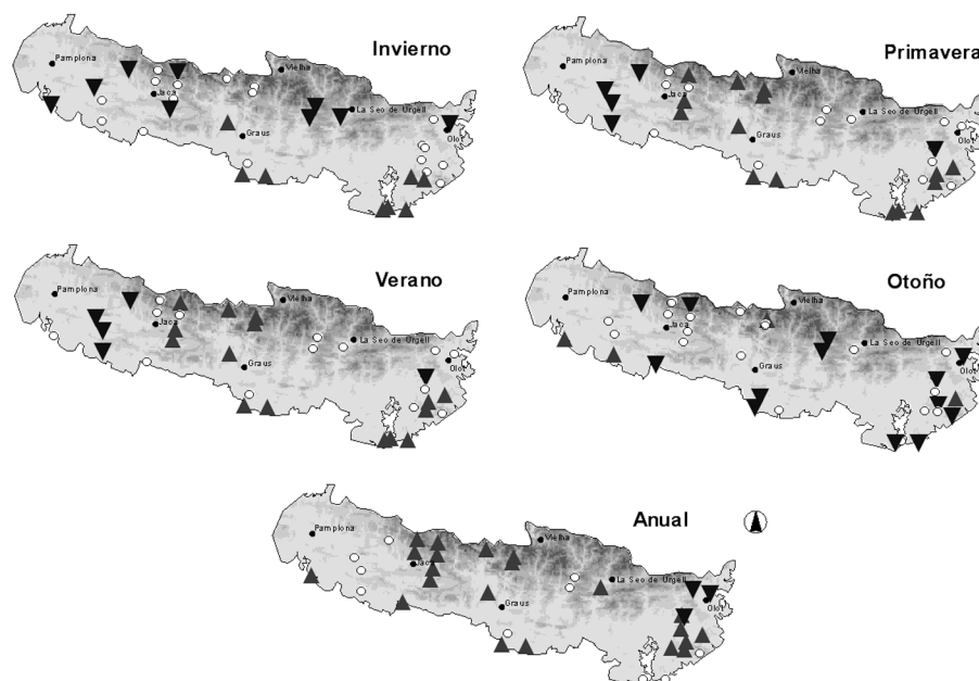
Figura 13. Distribución espacial de las tendencias en la duración máxima de las rachas secas (1951-2001). Triángulos: tendencia positiva y significativa. Triángulos invertidos: tendencia negativa y significativa. Círculos: Tendencia no significativa.
