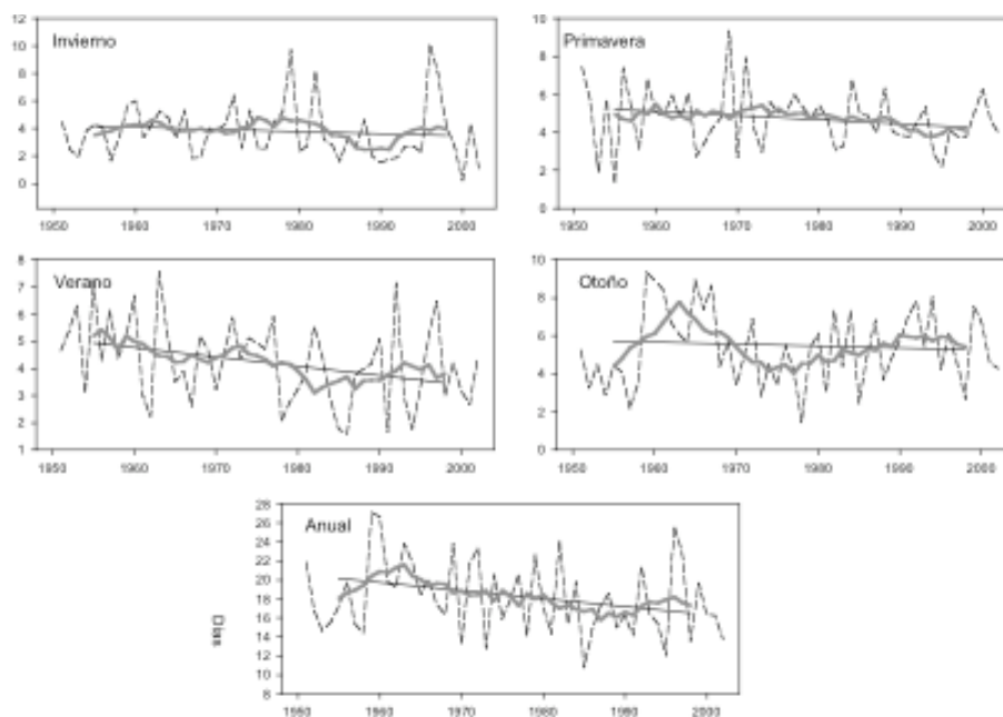
Figura 6. Evolución del número de días con un volumen de precipitación superior al 95 percentil estacional y anualmente (1951-2001). Línea negra discontinua (número de días observado), línea gris (filtro de 9 años). La línea de tendencia se obtiene mediante el ajuste por mínimos cuadrados a partir de los datos filtrados.
