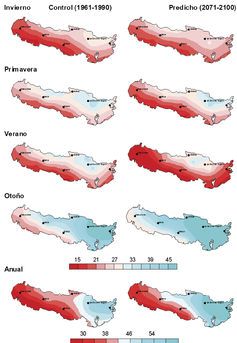
Figura 16. Distribución espacial del promedio del máximo evento estacional y anual. Modelo RAO, SMHI. Periodo de control (1961-1990) y escenario A2 (2071-2100). Figure 16. Spatial distribution of average seasonal and annual maximum rainy day. Model RAO, SMHI. Control period (1961-1990) and scenario A2 (2071-2100).
