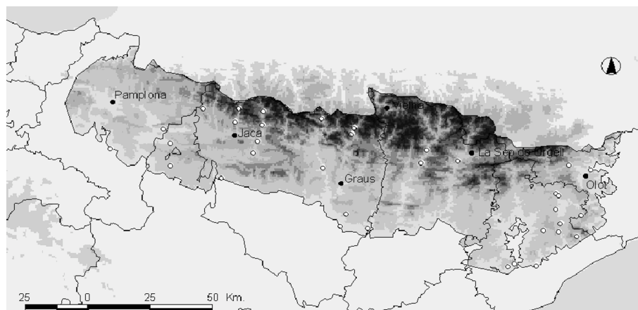
Figura 1. Área de estudio y distribución de los observatorios meteorológicos utilizados (puntos blancos).
