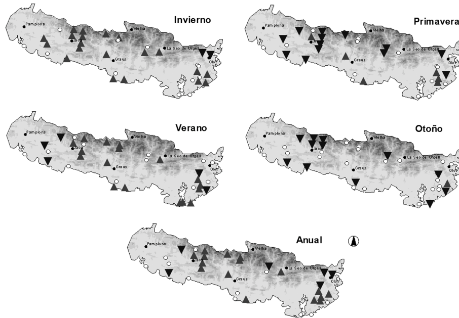
Figura 11. Distribución espacial de las tendencias en la duración media de las rachas secas (1951-2001). Triángulos: tendencia positiva y significativa. Triángulos invertidos: tendencia negativa y significativa. Círculos: Tendencia no significativa.
