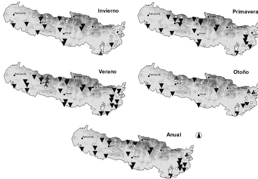
Figura 7. Distribución espacial de las tendencias en el número de días con un volumen de precipitación superior al 95 percentil estacional y anualmente (1951-2002). Triángulos: tendencia positiva y significativa. Triángulos invertidos: tendencia negativa y significativa. Círculos: Tendencia no significativa.
