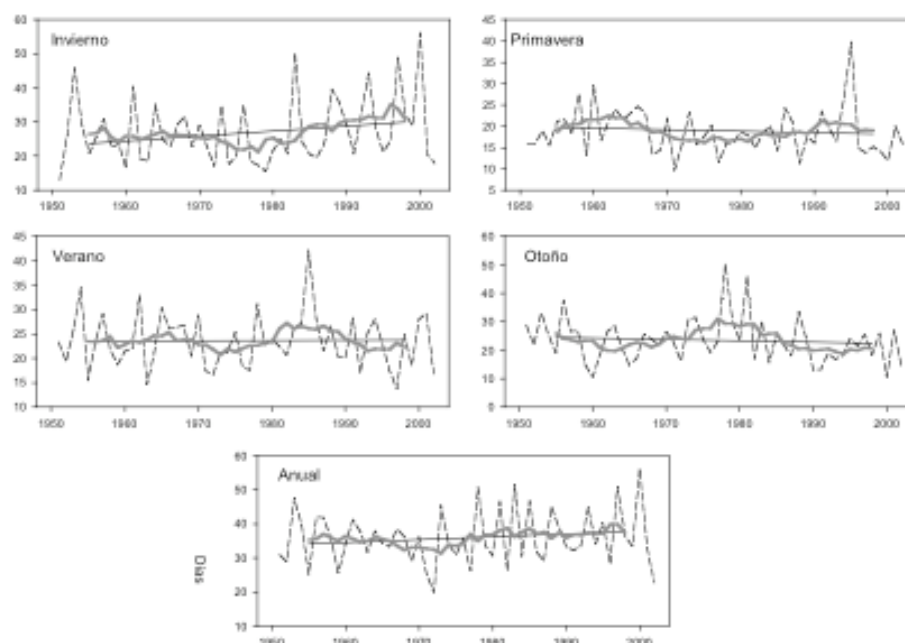
Figura 12. Evolución de la duración máxima de las rachas secas (1951-2001). Línea negra discontinua (promedio de duración de las rachas secas), línea gris (filtro de 9 años). La línea de tendencia se obtiene mediante el ajuste por mínimos cuadrados a partir de los datos filtrados. Figure 12. Evolution of the seasonal and annual duration of maximum dry spells (1951-2001). Black line (observed number of days), gray line (low pass filter of 9 years). The trend line has been obtained by means of regression analysis by means of filtered data.
