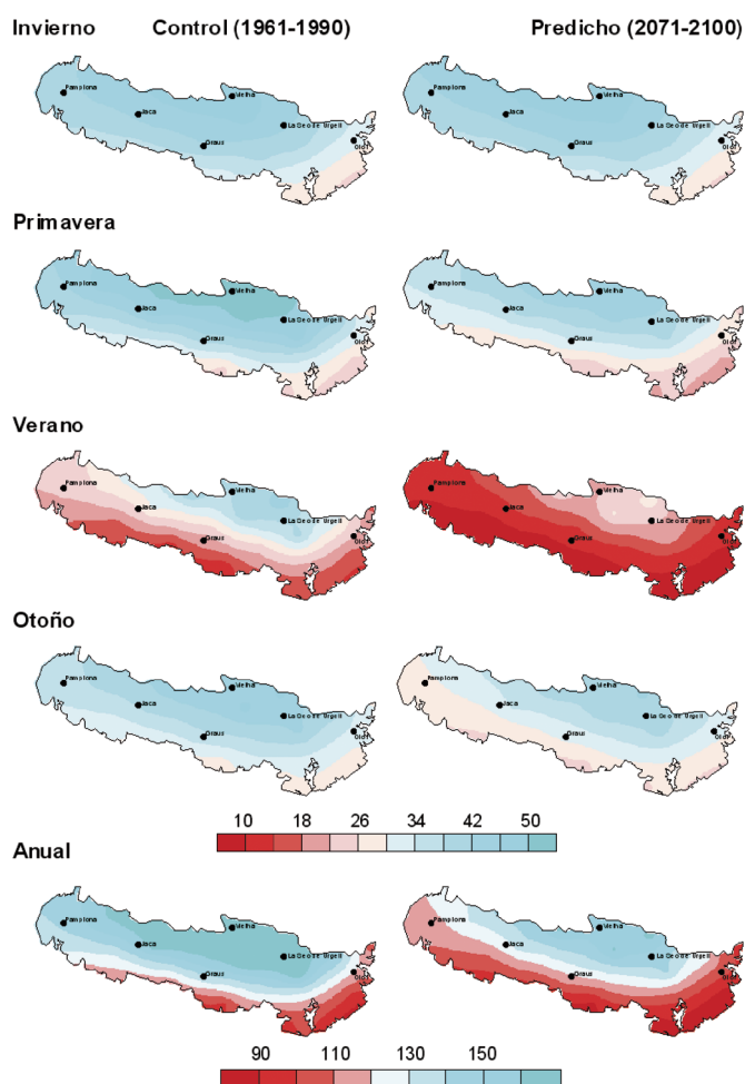
Figura 15: Distribución espacial del promedio de días de precipitación. Modelo RCAO, SMHI. Periodo de control (1961-1990) y escenario A2 (2071-2100).
