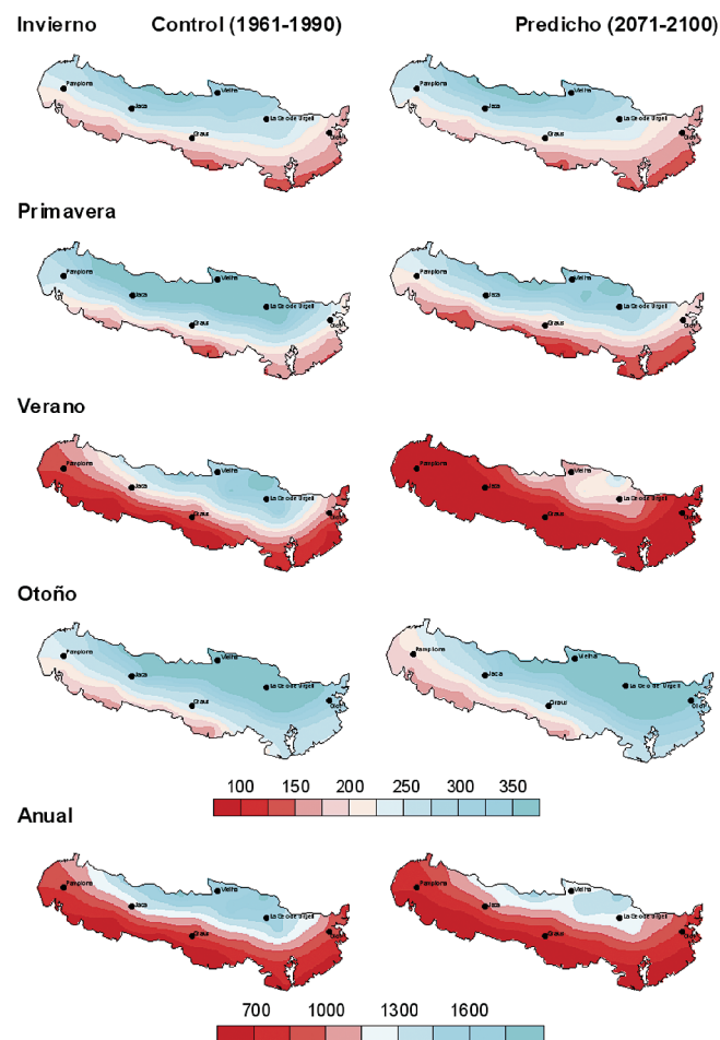
Figura 14: Distribución espacial del volumen de precipitación (mm.). Modelo RCAO, SMHI. Periodo de control (1961-1990) y escenario A2 (2071-2100). Figure 14. Spatial distribution of precipitation amount (mm.). Model RCAO, SMHI. Control period (1961-1990) and scenario A2 (2071-2100).
