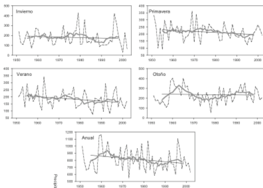
Figura 2. Evolución de los volúmenes estacionales y anuales de precipitación (1951-2001). Línea negra discontinua (precipitación observada), línea gris (precipitación filtrada con un filtro de 9 años). La línea de tendencia se obtiene mediante el ajuste por mínimos cuadrados a partir de los datos filtrados.
