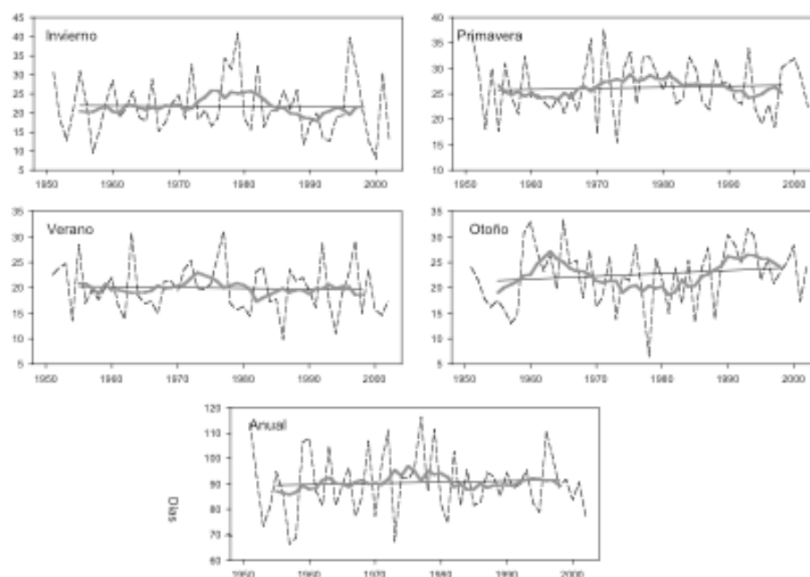
Figura 4. Evolución del número de días de precipitación estacional y anual (1951-2001). Línea negra discontinua (número de días observado), línea gris (filtro de 9 años). La línea de tendencia se obtiene mediante el ajuste por mínimos cuadrados a partir de los datos filtrados.
