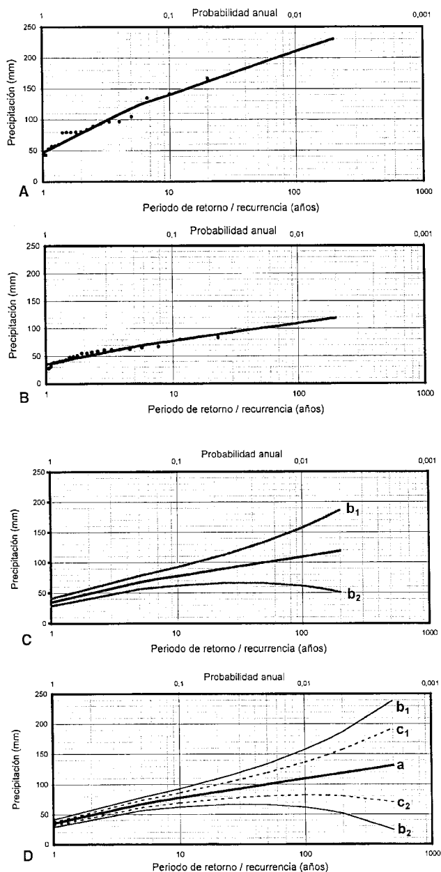
Figura 2. Precipitación correspondiente a diferentes períodos de retorno. A. Estación meteorológica de La Sarra (alto Gállego). B. Estación meteorológica de Jaca. C. Estación meteorológica de Jaca, con inclusión de la banda de confianza al nivel de significación 90% ( b_1 , b_2 ). D. Estación meteorológica de Jaca, con inclusión de la misma banda de confianza para una serie teórica de 100 años ( c_1 , c_2 )
