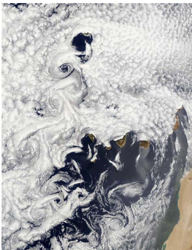
2. Canarias desde satélite
