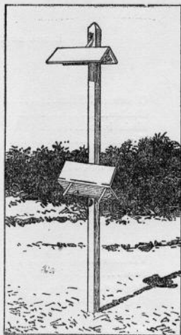
Fig. 4. — Estació composta de dos abrics senzills per a termòmetres de mínima situats a 1,50 m. i a 70 cm. d'altura.
