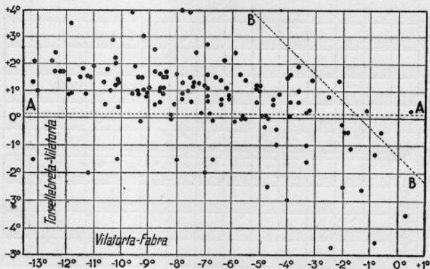
Fig. 9. — Correlació entre les diferències de temperatura mínima diària (Vilatorça minus Fabra) i les simultànies (Torrellebreta minus Vilatorça), per als mesos de novembre a març. La significació de les lletres és anàloga a la de la fig. 6.
