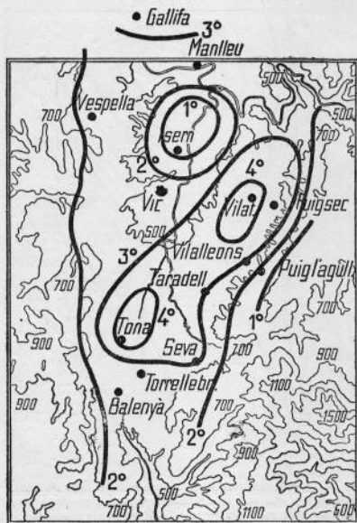
Fig. 12. — Temperatures mínimes promigues, durant els mesos d'hivern, els dies que la mínima de Vilatorça no ha arribat a ésser 3^{\circ} més baixa que la de l'Observatori Fabra. Corresponen a temps revolt, de vent, de núvols o de boira.
