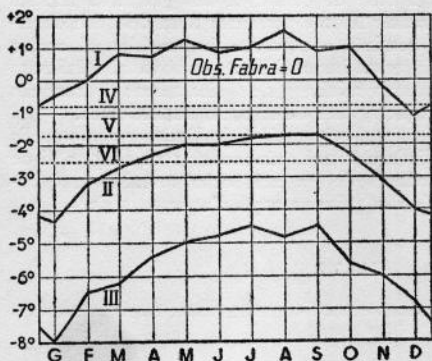
Fig. 1. — Diferències (Vilatorta minus Fabra) entre els promitjos mensuals de les temperatures màximes, mitges i mínimes diàries. I. Diferència entre les màximes observades. — II. Diferència entre les mitges observades. — III. Diferència entre les mínimes observades. — IV. Diferència calculada en la hipòtesi d'un gradient uniforme de 0,5° per 100 m. — V. Diferència calculada en la hipòtesi d'un gradient adiabàtic. — VI. Diferència efectiva entre les temperatures mitges de l'any.
