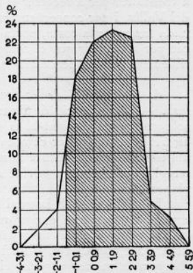
Fig. 14. — Freqüència, per 100, de les diferències entre les temperatures màximes (Vilatorça minus Fabra), per intervals d'1° i per als mesos de juny, juliol i agost dels anys 1924-25. La regió ombrejada correspon a la calor anòmla de les migdiades a Vilatorça.
