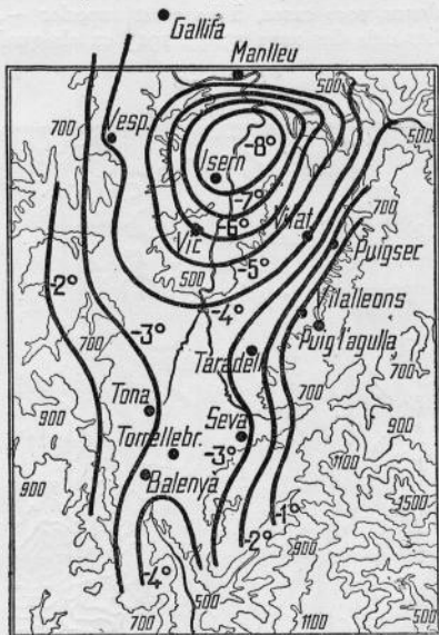
Fig. 11. — Temperatures mínimes promitges, durant els mesos d'hivern, els dies que la mínima de Vilatorra ha estat 7^{\circ} o més més per sota de la de l'Observatori Fabra. Corresponen a matinales subsegüents a nits de calma i cel seré.
