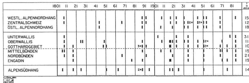
Figura 10. "Calendario" de la actividad avalanchosa catastrófica en los Alpes Suizos (1800-1985). Cada barra negra marca un evento catastrófico en la región indicada. Los periodos de retorno medios se tabulan en el margen derecho. (Extraída de Föhn, 1992).
