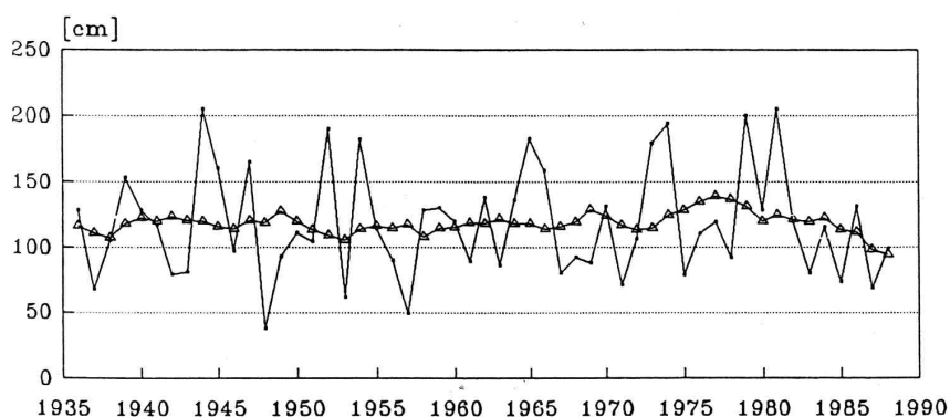
Figura 8. Espesor de nieve el 1 de Enero en Weissfluhjoch (2540 m) y media solapada de 11 años. (Extraída de Föhn, 1992). Figure 8. Snow depth yearly at the 1st January on Weissfluhjoch (2540 m) and 11-year overlapping means. (Extracted from Föhn, 1992).
