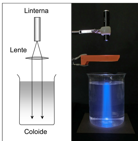
Figura 2. El coloide de poliestireno se ilumina desde arriba con una linterna de luz blanca, cuya luz ha sido parcialmente colimada con una lente convergente. La luz esparcida es de color azulado.
