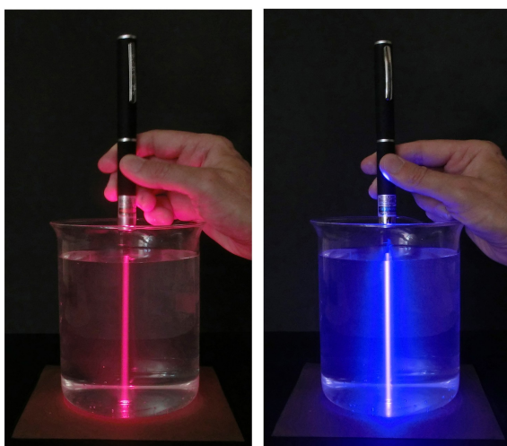
Figura 1. Un coloide de poliestireno se ilumina desde arriba con un láser rojo (izquierda) y con un láser violeta (derecha). La luz violeta sufre un esparcimiento mayor que la luz roja.
