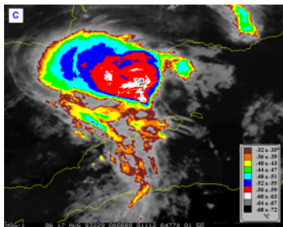
Fig. 5.- Satélite MSG-1, 17 de Agosto de 2003, canal de 10,7 \mu\text{m} a las 8 UTC.
