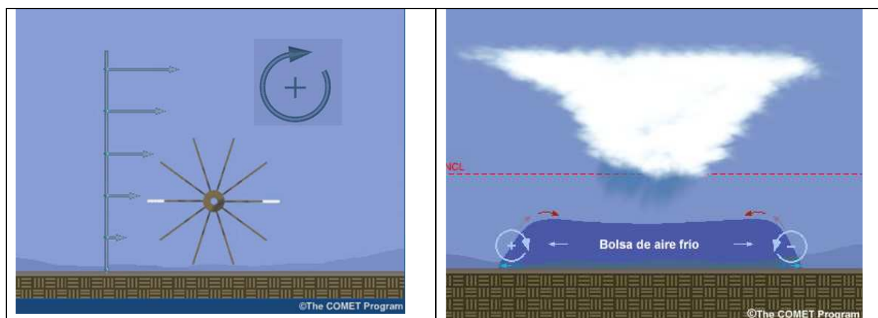
Figura 2.6. Izda: Cizalladura vertical de viento promotora de vorticidad de eje horizontal. Dcha: vorticidades opuestas generadas a ambos lados de los bordes de una bolsa de aire frío. Fuente: The Comet Program
