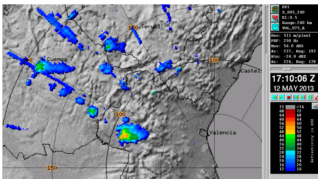
Figura 4.5: PPI de Reflectividad, que insinúa la presencia de un gancho.
