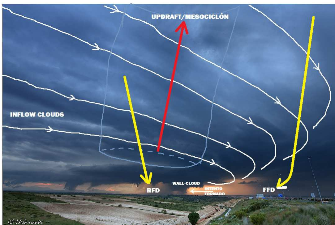
Figura 4.4: Foto de la supercélula de Madrid, del 6 de mayo de 2011, con identificación de elementos básicos. Fuente: J.A. Quirantes, 2012. http://foro.tiempo.com/supercelula-americana-a-25-km-de-la-puerta-del-sol-madrid-6mayo2011-t131853.0.html
