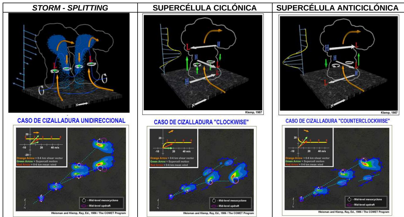
Figura 2.15. Tipos de cizalladura y estructuras convectivas resultantes.
