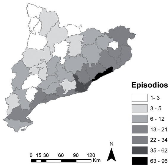
FIG. 1: Mapa de comarcas afectadas por inundaciones desde 1981 al 2010.
