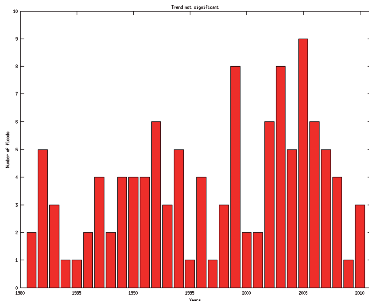
FIG. 6: Evolución anual del número de inundaciones extraordinarias en Cataluña para el periodo 1981-2010. No se observa ninguna tendencia significativa al 95%.
