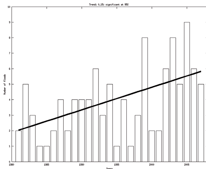
FIG. 7: Evolución anual del número de inundaciones extraordinarias en Cataluña para el periodo 1981-2007. Se observa una tendencia significativa al 95% de 0.15 inundaciones/año.
