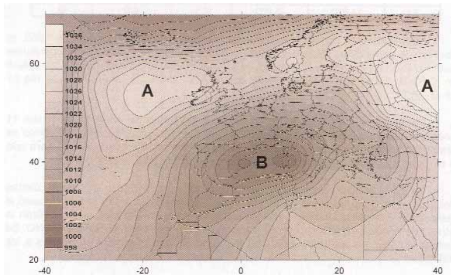
Figura 5. Mapa isobárico del 15 de enero de 1885 Fuente de datos: Met Office – Hadley Center
