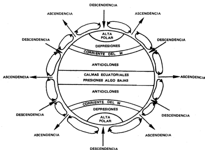
Figura 1: Esquema de la circulación atmosférica.
