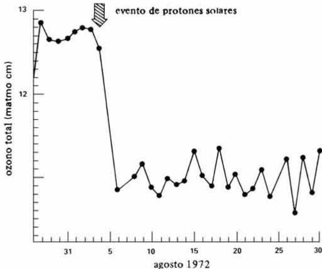
Figura 23. Reducción del ozono por efecto de las partículas solares sobre la atmósfera en las altas altitudes. (De acuerdo con D. Heath).
