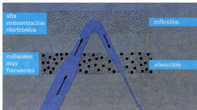
Figura 16. a) Si la concentración de electrones es muy elevada a gran altitud las ondas de radio son reflejadas, en tanto que si la concentración elevada ocurre a baja altitud esas ondas son absorbidas. Para radiación de frecuencia muy elevada no hay suficientes electrones para que se efectúe la reflexión, en tanto que para frecuencias bajas la absorción es muy fuerte. b) Se ilustra la alteración del rango de frecuencias utilizables para las comunicaciones entre Londres y Halifax (Canadá) durante un mínimo solar (diciembre de 1954) y el máximo solar siguiente (diciembre de 1958). Las zonas blancas indican las frecuencias utilizables, las zonas azules y grises indican frecuencias limitadas por reflexión y absorción respectivamente. Las frecuencias inferiores a los MHz no fueron accesibles por haber sido reflejadas por la capa E de nuestra atmósfera. c) Durante una tormenta ionosférica la frecuencia límite para la reflexión decrece en tanto que la frecuencia límite para la absorción crece. Los diagramas muestran cómo esas modificaciones reducen la banda de frecuencia disponibles para las comunicaciones, y se pone en evidencia cómo los efectos de una tormenta magnética son más severos en el mínimo de actividad solar (de acuerdo con J. A. Ratcliffe).
