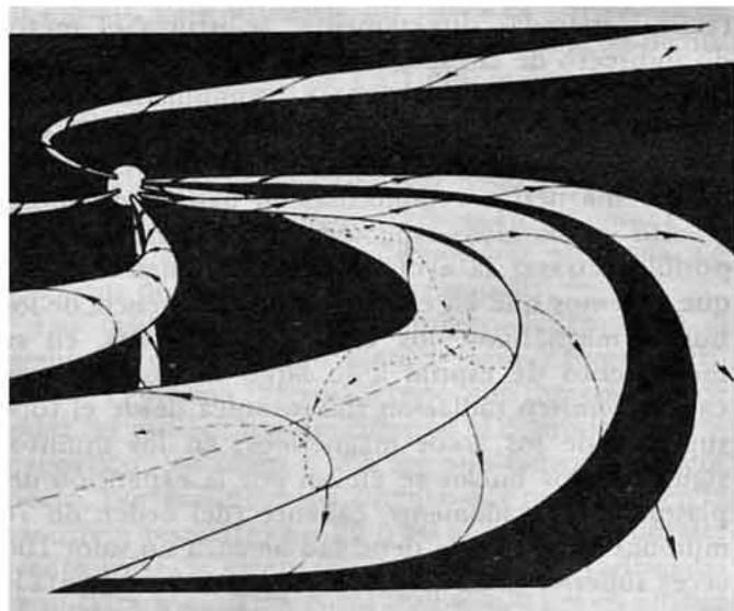
Figura 21. Esquematización de los "tubos" de campo magnético (tubos de Arquímedes) en que se concentran las líneas de campo magnético interplanetario.
