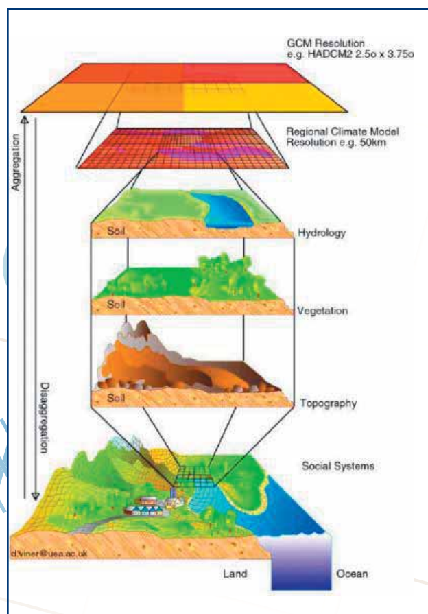
Fig. 4.- Las diferentes técnicas de regionalización o reducción de escala (downscaling) adaptan las salidas de los modelos globales AOGCMs a las características fisiográficas (topografía, vegetación, etc) de una determinada región (fuente: Climate Research Unit, 2000)
