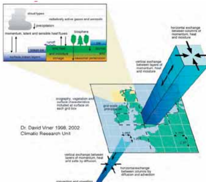
Fig. 1. - Los modelos de circulación general acoplados de atmósfera y océano en la discretización de las ecuaciones termo-hidrodinámicas de la atmósfera y océano. La figura representa los intercambios verticales y horizontales (de momento, calor y humedad) en la atmósfera y (de momento, calor y salinidad) en el océano. También se representan las características fisiográficas de la superficie terrestre y la parametrización de los procesos subrejilla (fuente: D. Viner, Climatic Research Unit, 2000).
