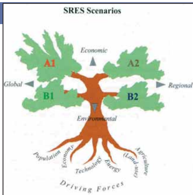
Fig. 3.- Los escenarios de emisión SRES (IPCC Special Report on Emission Scenarios) abarcan el conjunto de las principales fuerzas determinantes: demografía, economía, tecnología, energía, uso del suelo y agricultura. También distinguen entre las soluciones globales o regionales al crecimiento económico y entre políticas que priorizan el medio ambiente o el crecimiento económico (fuente: IPCC, 2000).
