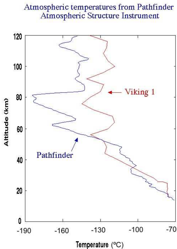
Figura 9.- Perfil térmico vertical de la atmósfera de Marte medido con la sonda espacial Viking 1 (en rojo) y con la Pathfinder (en azul). © NASA.
