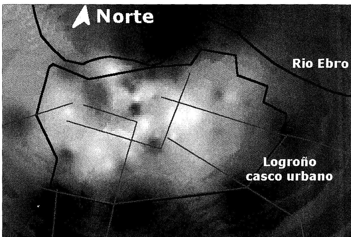
Fig.4 Modelo de la distribución térmica relativa en la ciudad de Logroño
