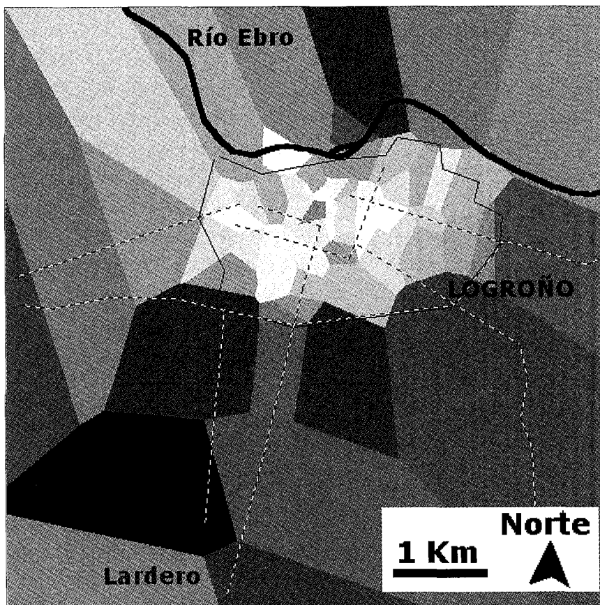
Fig.3 Distribución térmica relativa en la ciudad de Logroño interpolada según polígonos de Thiessen/Voronoi
