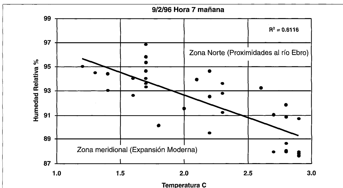
Fig.5 Relación entre la temperatura y humedad relativa
