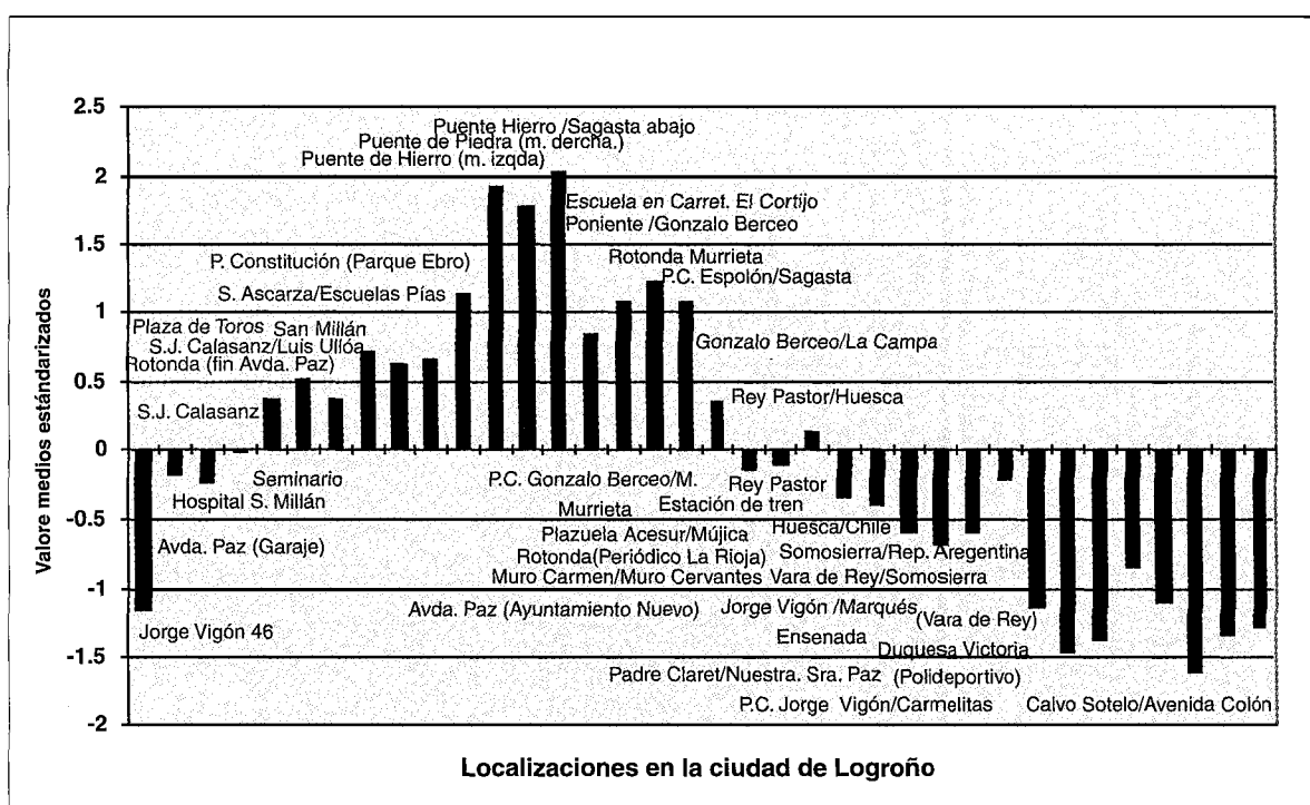
Fig.6 Diferenciación de la humedad relativa (valores medios estandarizados) en el microclima urbano
